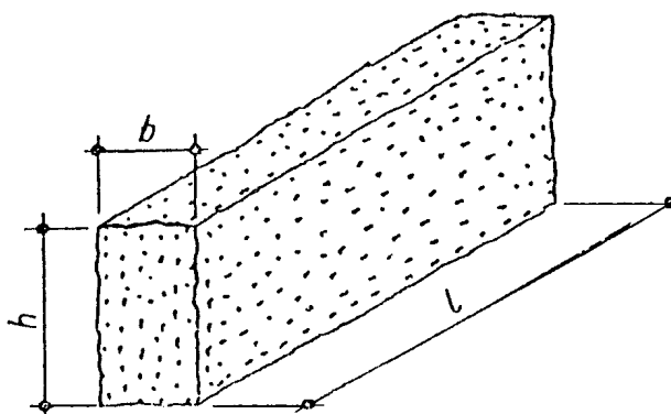
Rys. 6. Krawężnik - (opornik) drogowy rodzaju B
