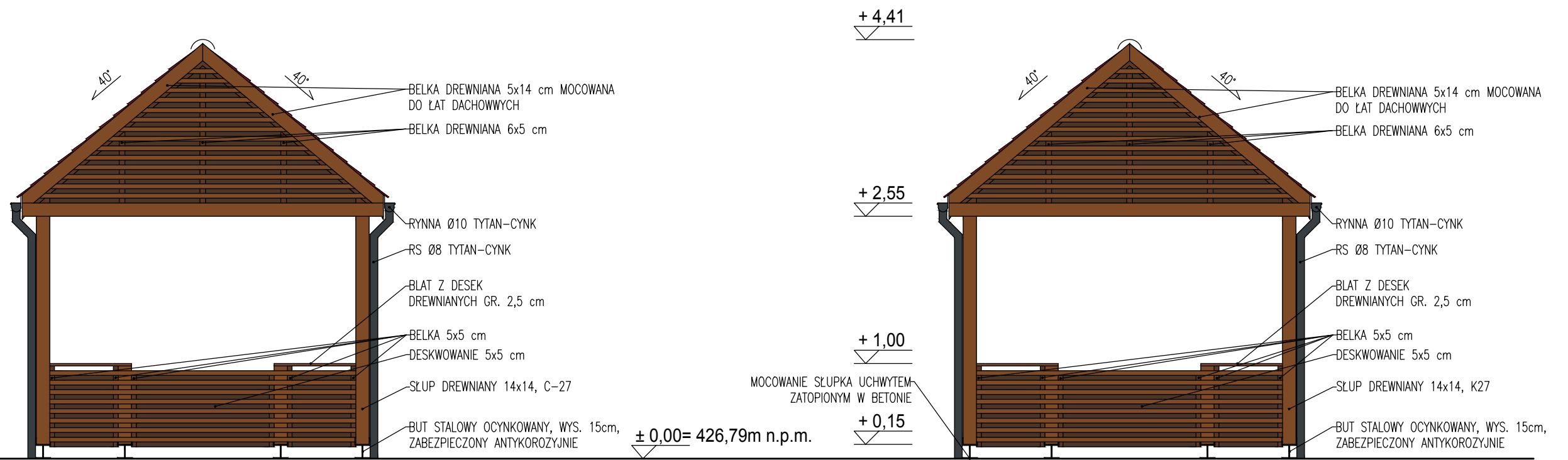
ELEWACJA PÓŁNOCNA I PÓŁDNIOWA
