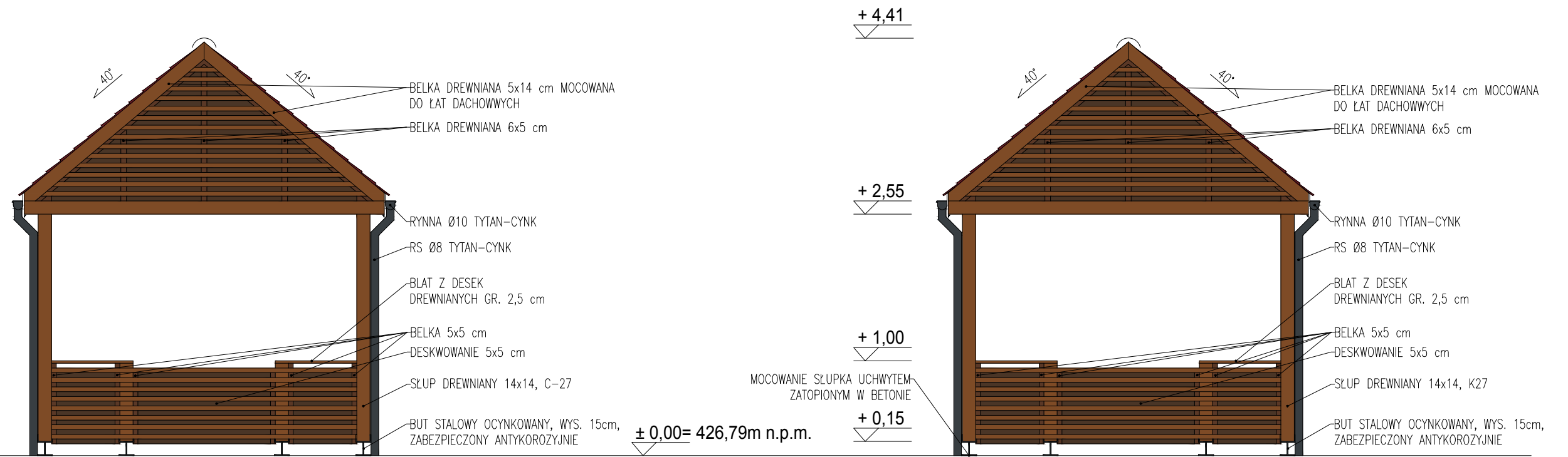
ELEWACJA PÓŁNOCNA I POŁUDNIOWA
