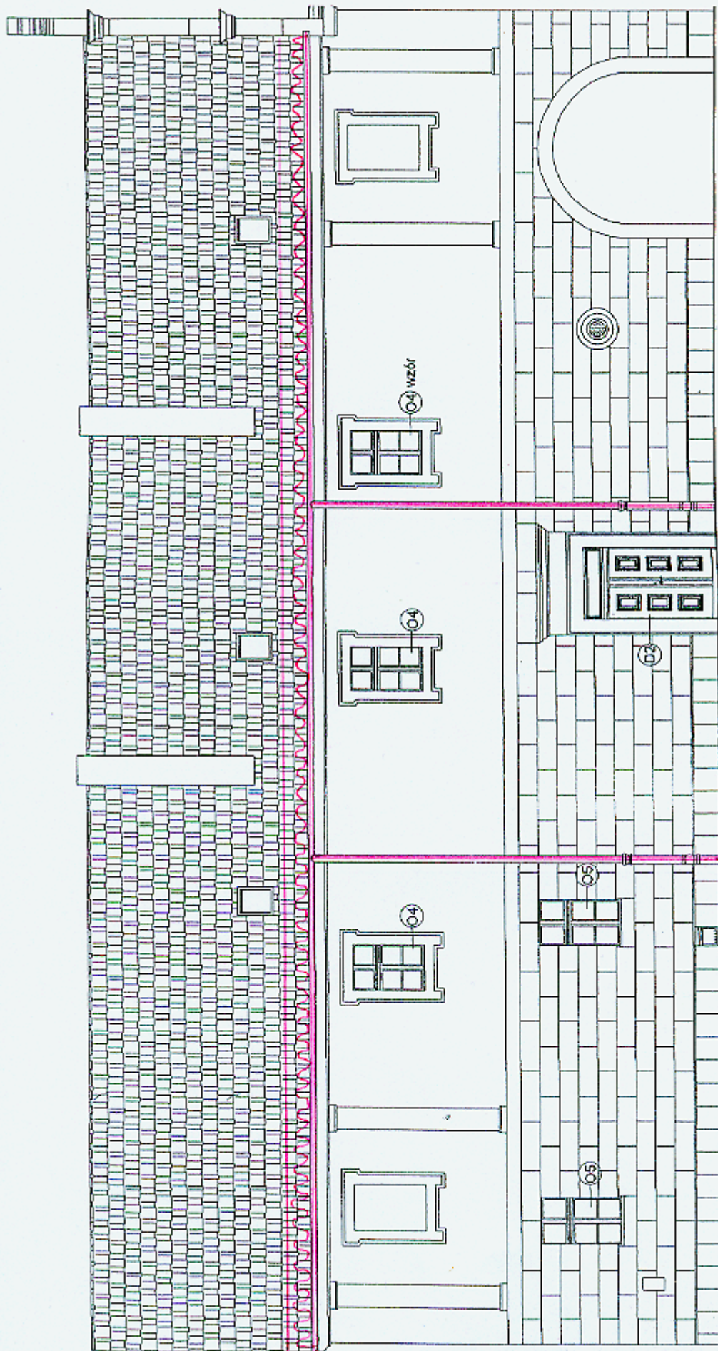
KAMIENICA NR 7 - ELEWACJA BOCZNA
