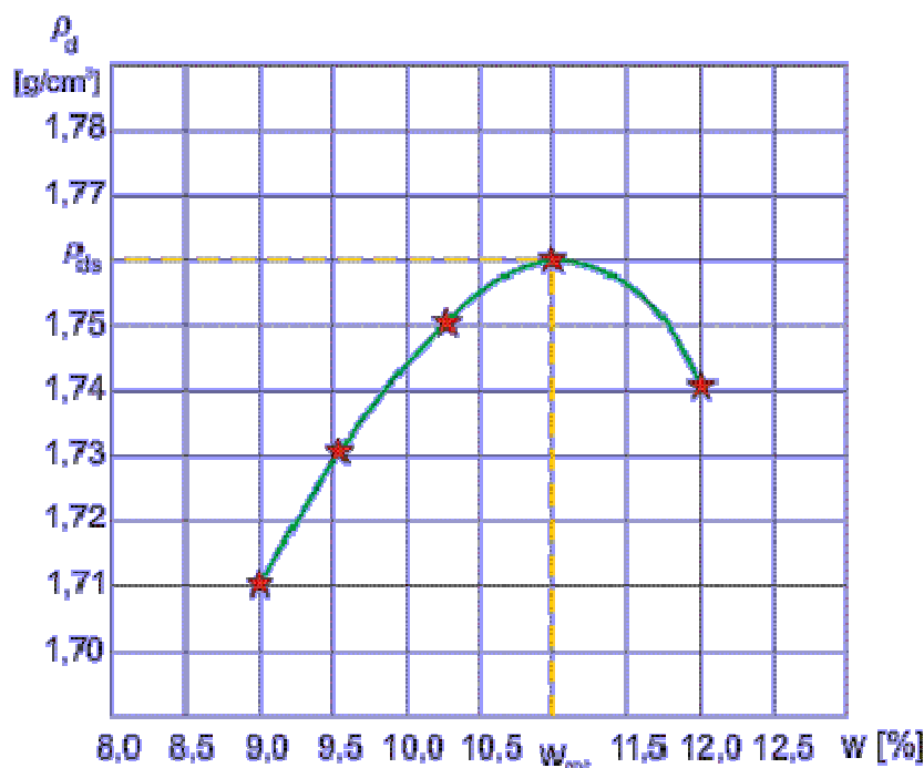
Rys. 4. Krzywa zagęszczalności gruntu
