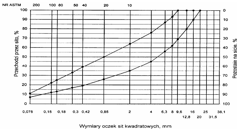
Rys. 3. Krzywe graniczne uziarnienia mieszanki mineralnej BA od 0 do 8mm, od 0 do 6,3 mm do warstwy ścieralnej nawierzchni drogi o obciążeniu ruchem KR1 lub KR2
