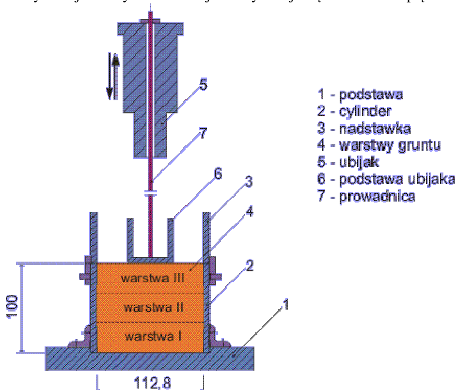
Rys. 3. Schemat aparatu Proctora
