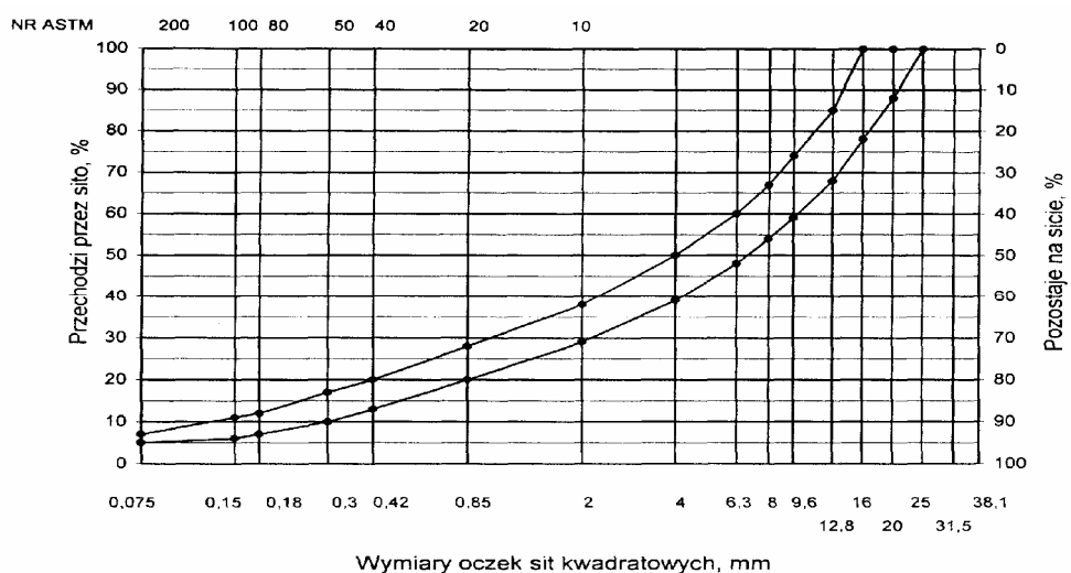
Rys. 5. Krzywe graniczne uziarnienia mieszanki mineralnej BA od 0 do 20 mm (mieszanka o nieciąglym uziarnieniu) do warstwy ścieralnej nawierzchni drogi o obciążeniu ruchem od KR3 do KR6
