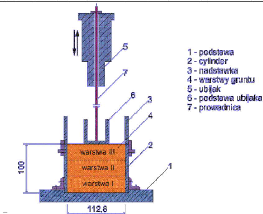
Rys. 3. Schemat aparatu Proctora
