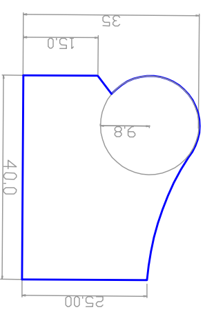
PRZEKRÓJ OBRZEŻA PŁASKOWOCWEGO 1:10
