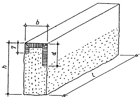
Krawężnik drogowy rodzaju B
