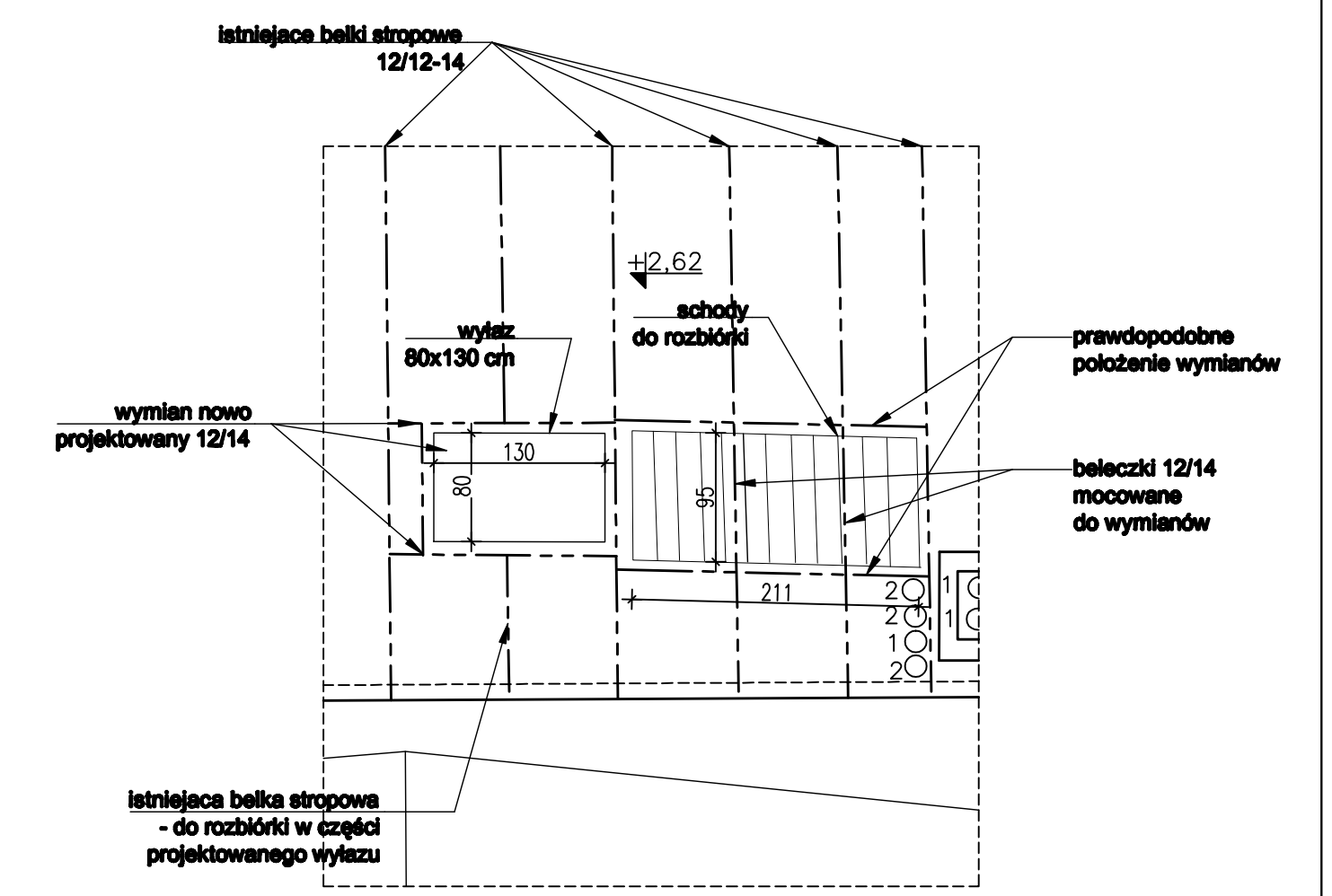
DETAL WYKONANIA WYŁAZU I STROPU W MIEJSCU SCHODÓW. SKALA 1:50
